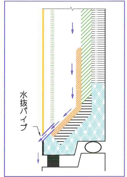
施工断面例
