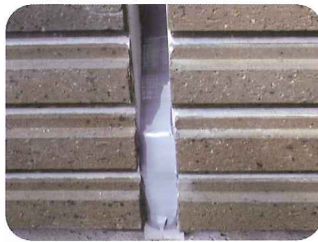
②下地シールの施工
